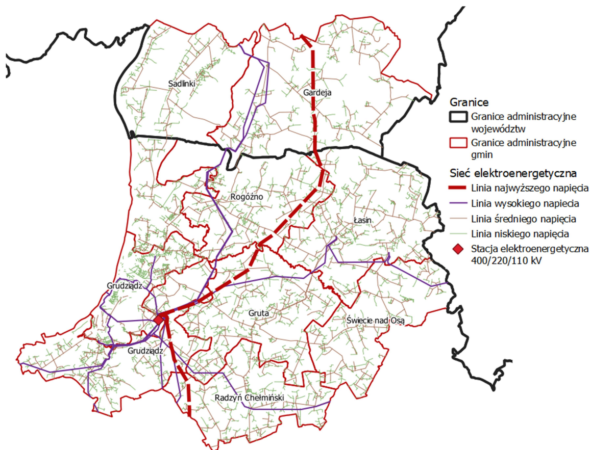
Rysunek 15: Sieć elektroenergetyczna na obszarze analizowanych JST
