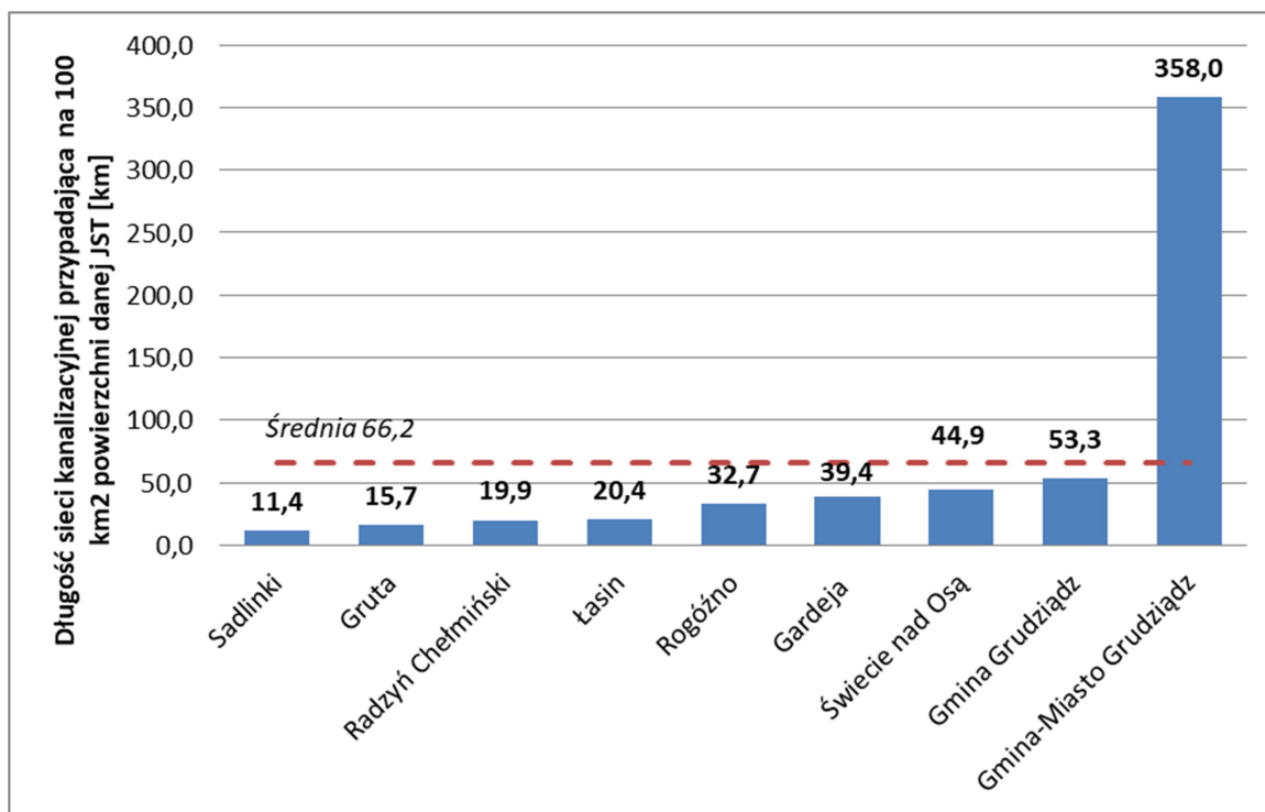
Wykres 37: Długość sieci kanalizacyjnej przypadająca na 100 km 2 powierzchni danej JST [km] w 2020 r.
