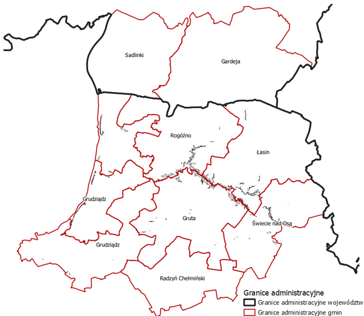
Rysunek 18: Tereny osuwiskowe i zagrożone ruchami masowymi na obszarze analizowanych JST
