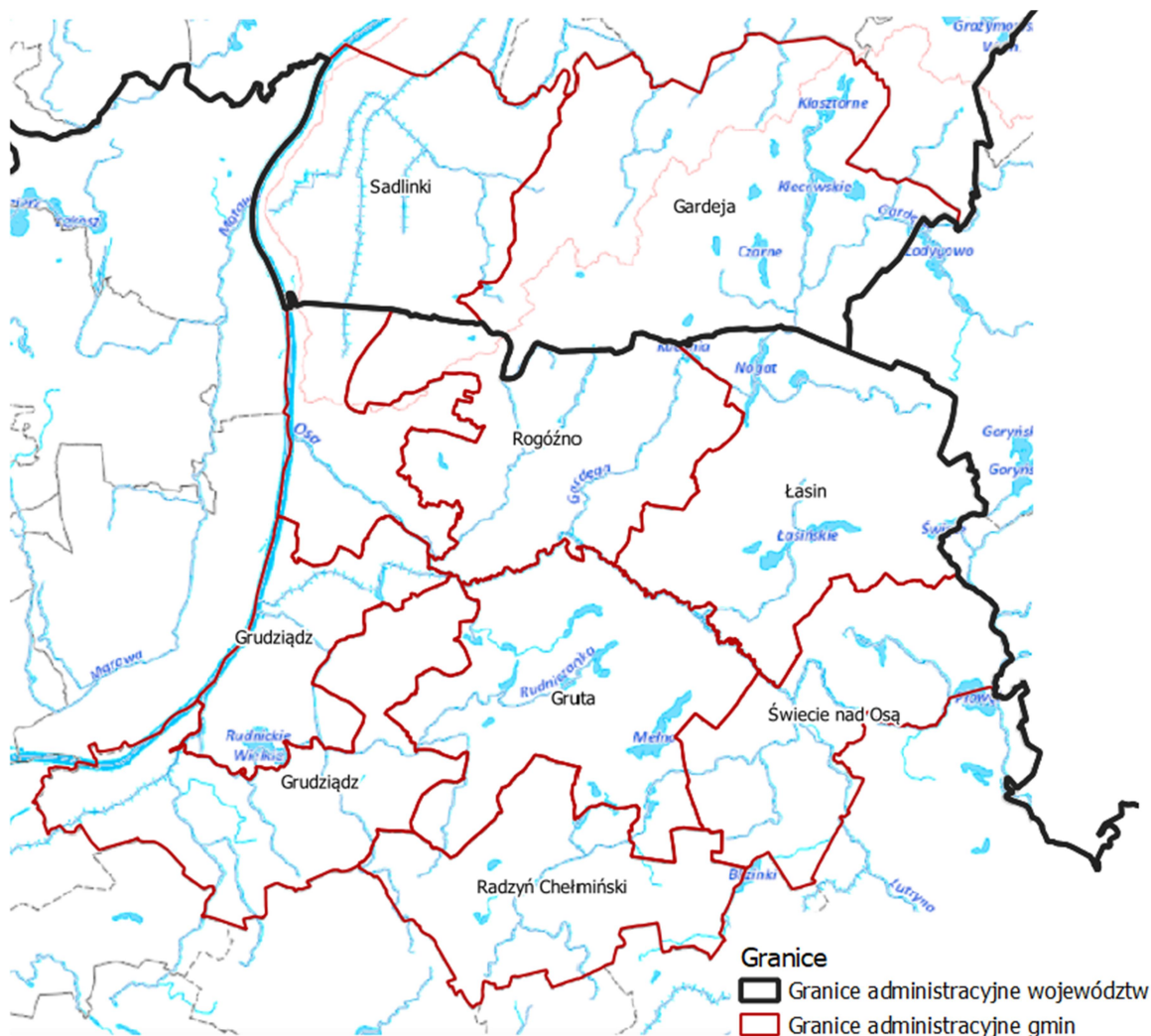
Rysunek 21: Podstawowa sieć hydrograficzna analizowanych JST
