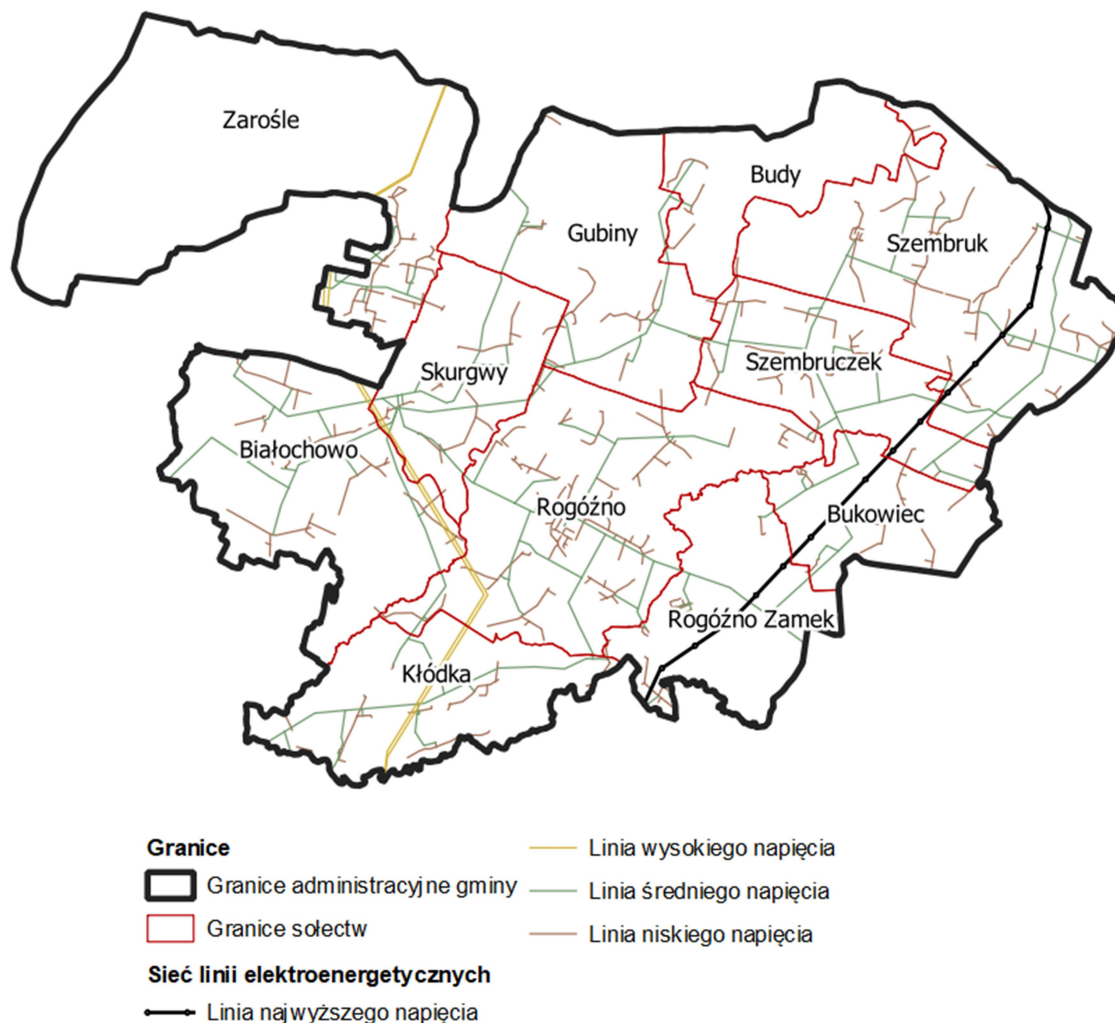
Rysunek 28: Przebieg sieci linii elektroenergetycznych w gminie Rogóżno
